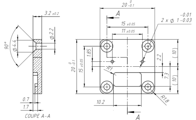
图5 A型编码器安装座 (参见表6)。
