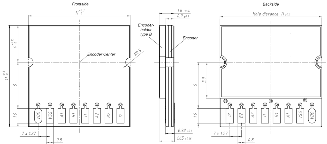
图3 在B型编码器安装座上的IT3402编码器的尺寸 (mm)。“编码器中心”必须相对码盘的“读数半径”位于中间位置 (图4)
