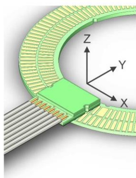
图1 XYZ轴坐标系。
