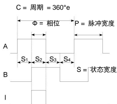
图2 A与B正交信号和参考信号的编码器输出信号。
