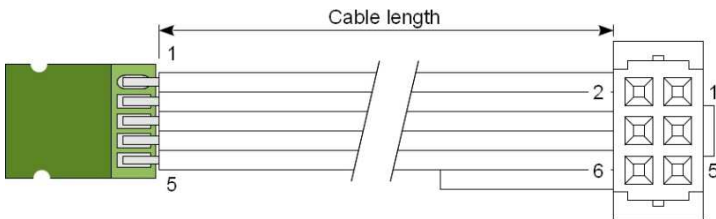
图6 带扁平电缆 (节距1.27 mm) 和6针接头DIN41651的编码器。
