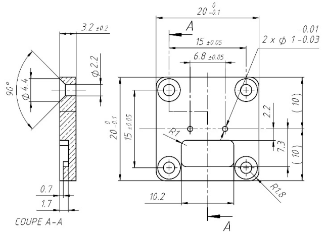
图5 A型编码器安装座的尺寸 (mm)。
