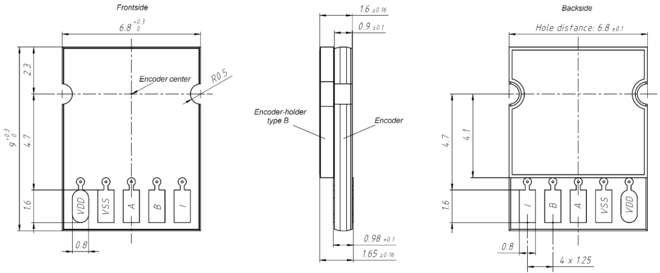
图3 在B型编码器安装座上的ID1102编码器的尺寸 (mm)。“编码器中心”必须相对读数头半径位于中间位置 (图4)。
