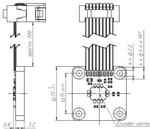
图7 在编码器A型安装座上的编码器尺寸 (mm) 和接头引脚编号, 编码器安装座连接扁平电缆 (节距1.27 mm) 和8针DIN41651接头。
