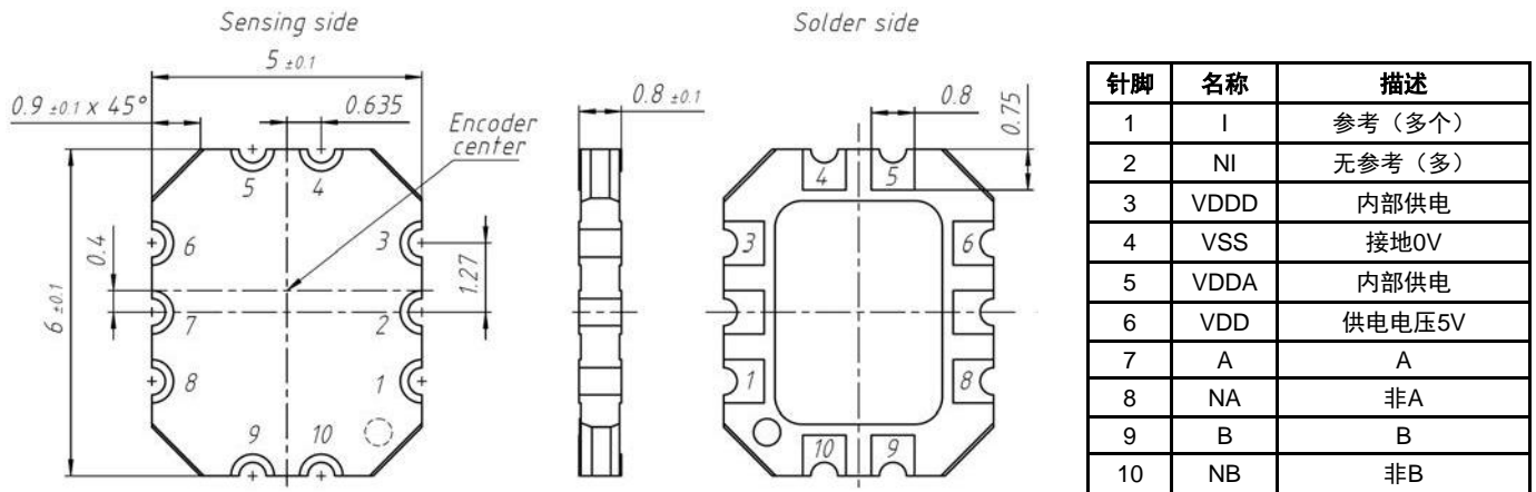
图3 编码器尺寸 (mm) 和引脚编号。必须相对尺带将“编码器中心”对中 (参见图4)。
