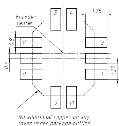
图6 推荐的布局。
