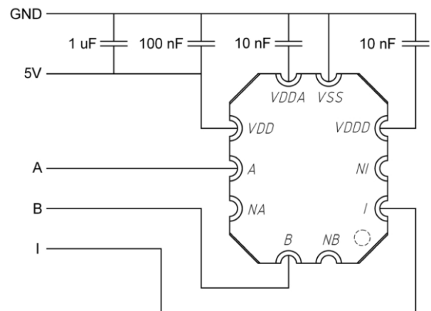
图5 推荐的线路图。电源滤波电容器应为1µF或更大。应确保100nF和2个10nF电容器位于该设备旁。为进行编程和线性化, 需要连接A、B和I。
